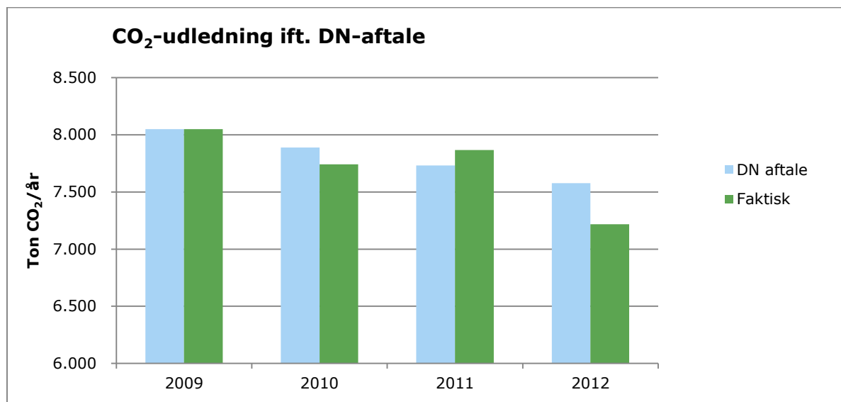
Figur 2. Udvikling i CO 2 -udledning for Faxe Kommune som virksomhed ift. DN Klimakommuneaftalen. Graddagekorrigeret varmeforbrug og med faste emissionsfaktorer for hhv. fjernvarme- og elforbrug.
