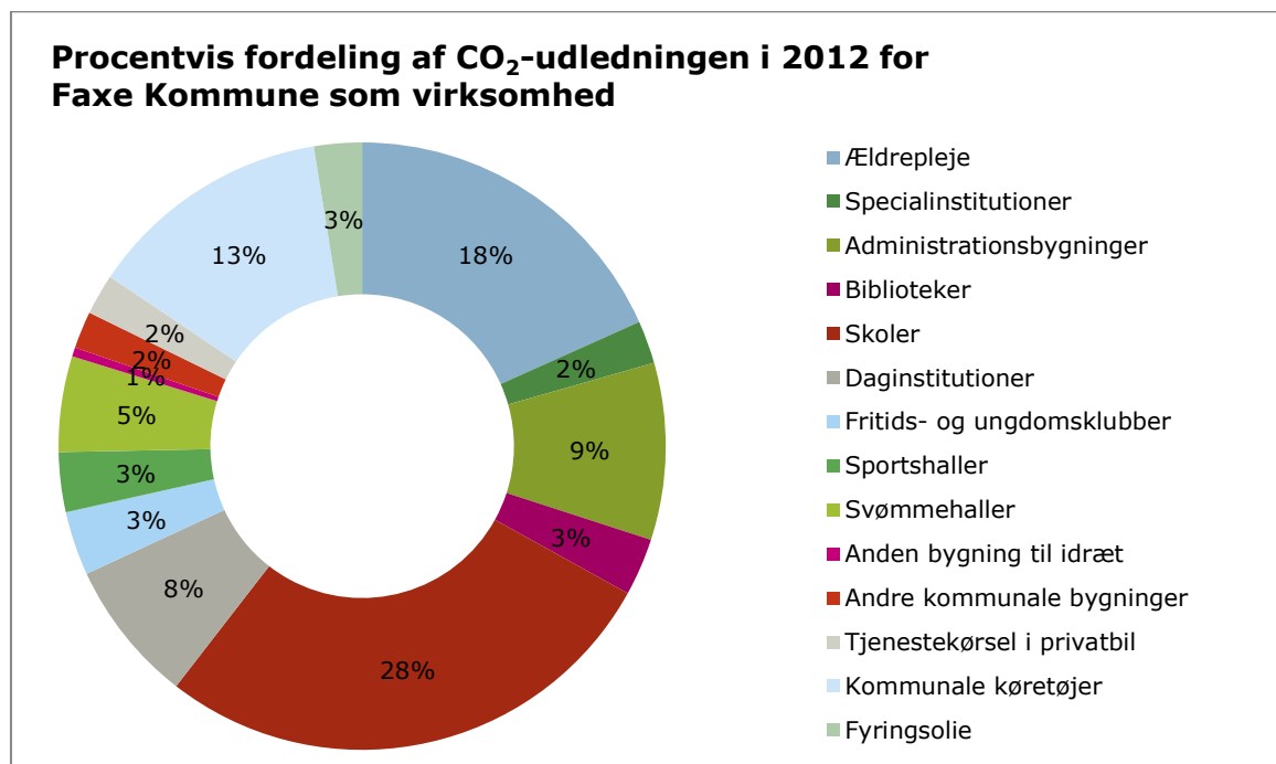
Figur 3. Den procentvise fordeling af CO 2 -udledningen. Graddagekorrigeret varmeforbrug og med fastlåste emissionsfaktorer for hhv. fjernvarme- og elforbrug.
